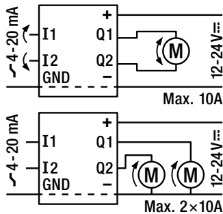
Function diagramm
