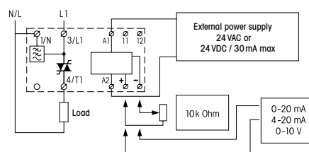
fig. 1. Wiring diagram
