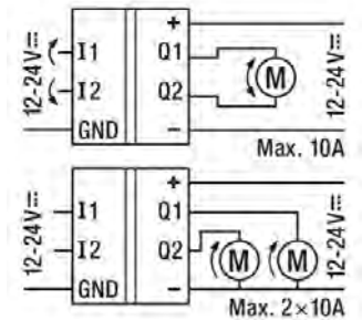
fig. 2. Function diagram
