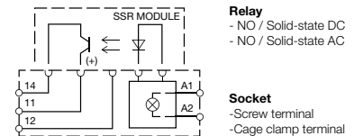
fig. 1. Wiring diagram
