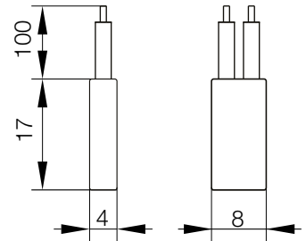
fig. 1. Dimension (mm)
