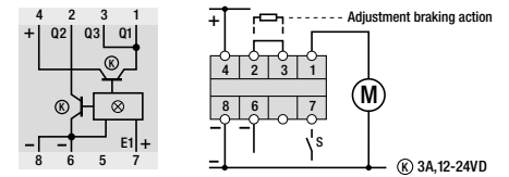
fig. 2. Function diagram
