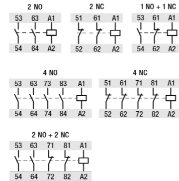
fig. 1. Wiring diagram
