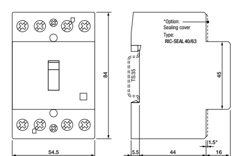
fig. 3. Dimensions (mm)
