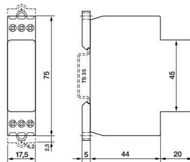
fig. 4. Dimensions (mm)
