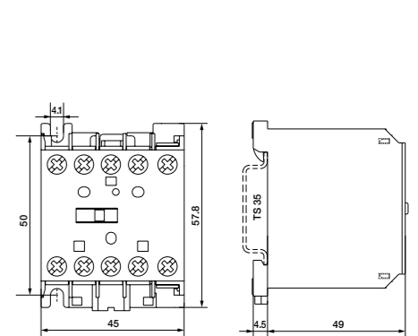
fig. 3. Dimensions (mm)
