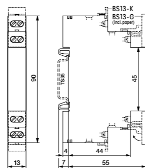
fig. 4. Dimensions (mm)
