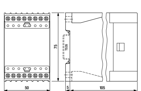
fig. 4. Dimensions (mm)
