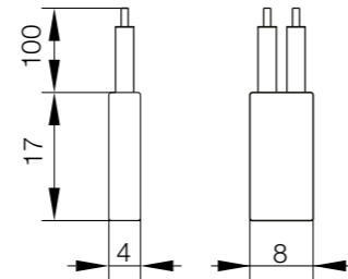
fig. 1. Dimensions (mm)
