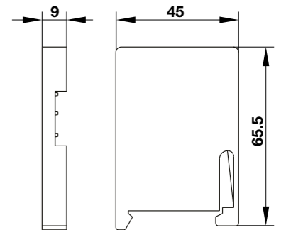
fig. 1. Dimensions (mm)
