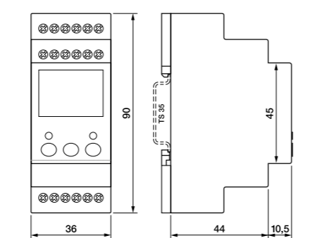
fig. 4. Dimensions (mm)
