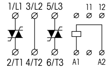
fig. 1. Wiring diagram
