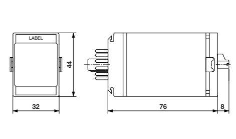
fig. 4. Dimensions (mm)
