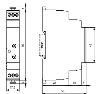
fig. 4. Dimensions (mm)
