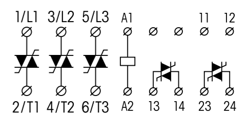
fig. 1. Wiring diagram
