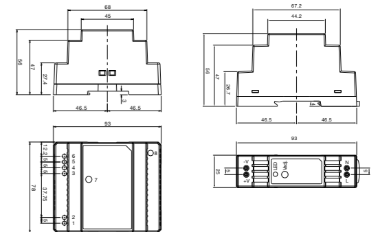
fig. 1. Dimensions (mm)
