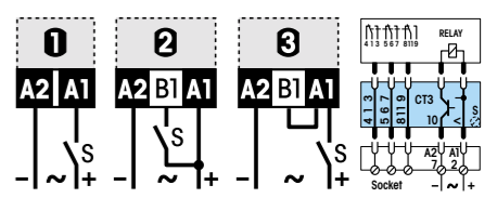
fig. 1. Wiring diagram
