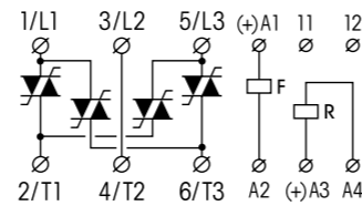
fig. 1. Wiring diagram
