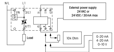
fig. 1. Wiring diagram
