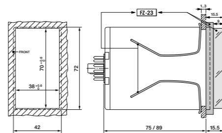
fig. 1. Dimensions (mm)
