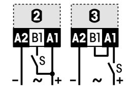
fig. 1. Wiring diagram
