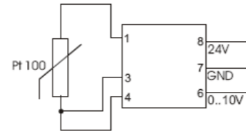
fig. 1. Wiring diagram
