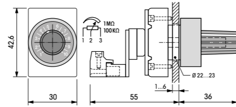
fig. 1. Dimensions (mm)
