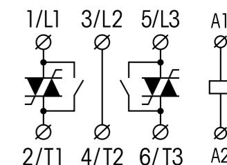
fig. 1. Wiring diagram
