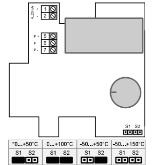
fig. 1. Wiring diagram
