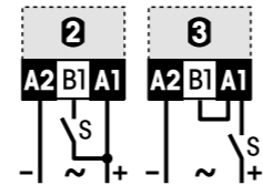
fig. 1. Wiring diagram
