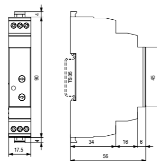
fig. 4. Dimensions (mm)
