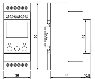
fig. 4. Dimensions (mm)
