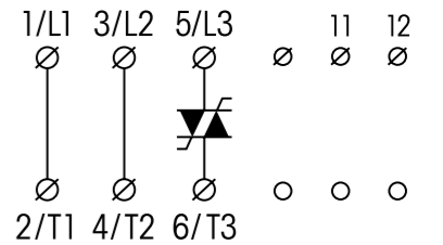
fig. 1. Wiring diagram
