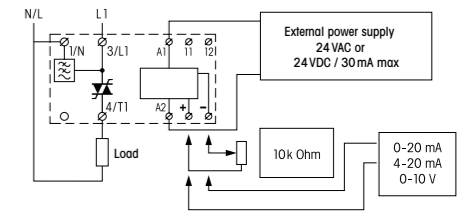
fig. 1. Wiring diagram
