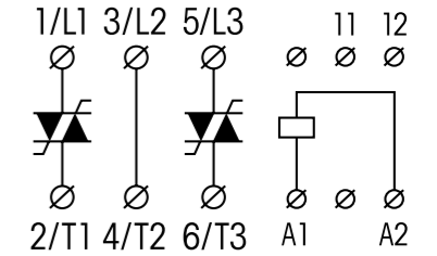
fig. 1. Wiring diagram
