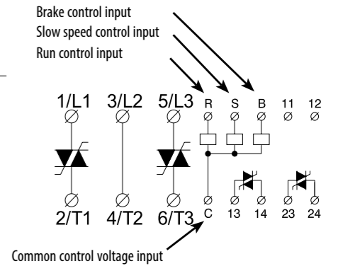
fig. 1. Wiring diagram
