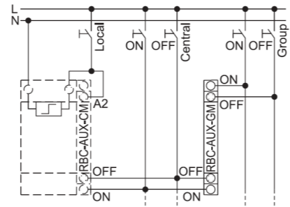
fig. 1. Wiring diagram
