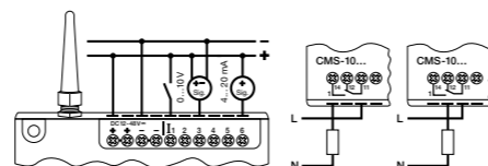
fig. 1. Wiring diagram
