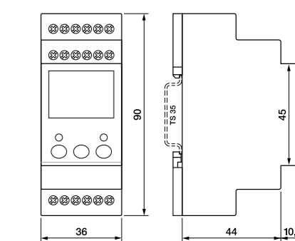
fig. 4. Dimensions (mm)
