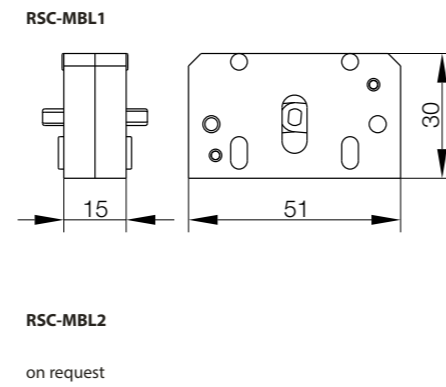
fig. 1. Dimensions (mm)
