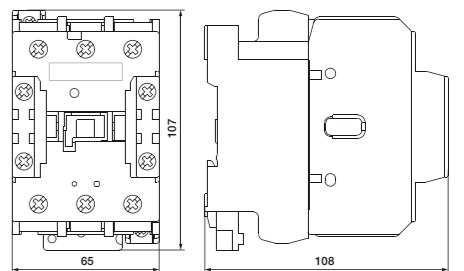
fig. 3. Dimensions (mm)
