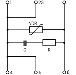
fig. 1. Wiring diagram
