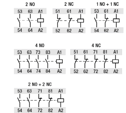
fig. 1. Wiring diagram
