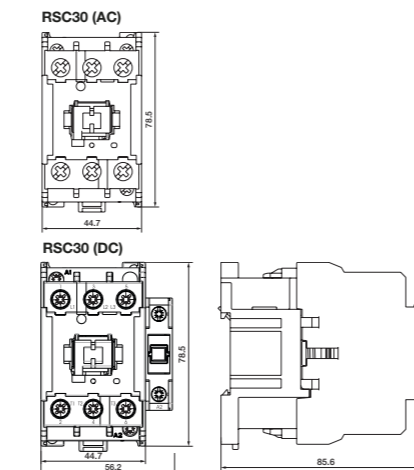
fig. 3. Dimensions (mm)
