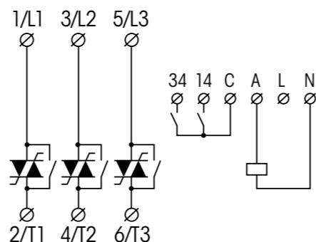
fig. 1. Wiring diagram
