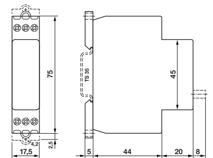
fig. 4. Dimensions (mm)
