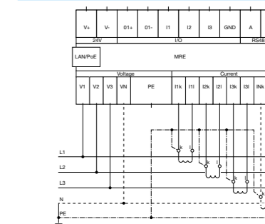
fig. 1. Wiring diagram
