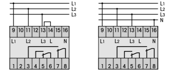
fig. 1. Wiring diagram
