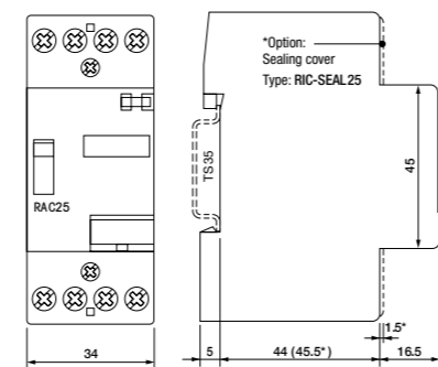
fig. 3. Dimensions (mm)
