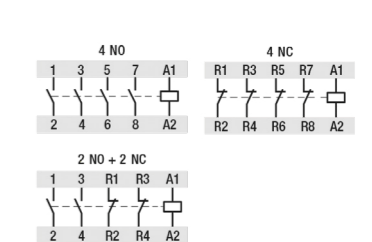
fig. 1. Wiring diagram
