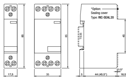
fig. 3. Dimensions (mm)
