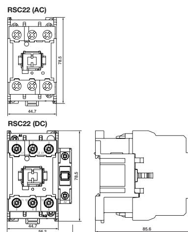
fig. 3. Dimensions (mm)
