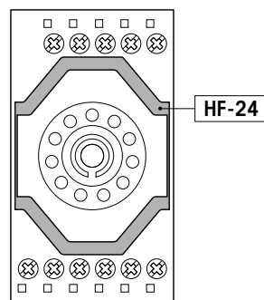
fig. 1. Dimensions (mm)
