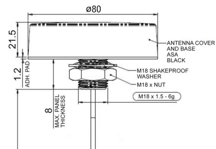
fig. 1. Dimensions (mm)
