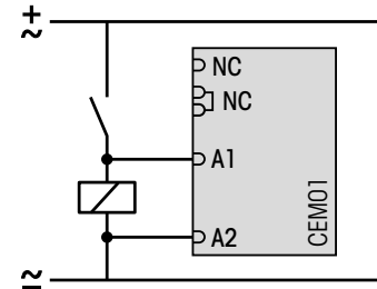
fig. 1. Wiring diagram
