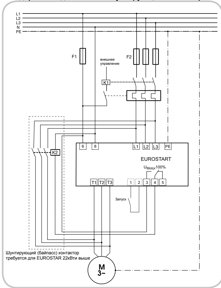
Стандартное подключение с шунтирующим контактором
