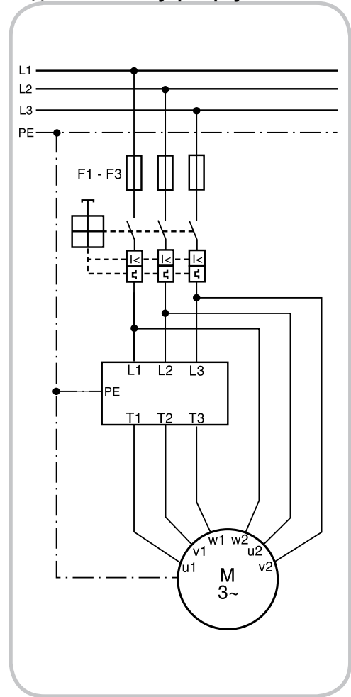
Подключение внутри треугольника
