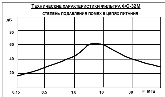
Рис.2. График АЧХ фильтра ФС-32М .
